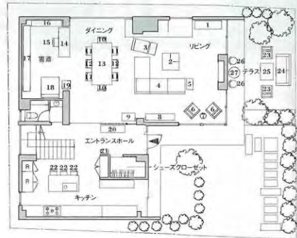
1F PLAN 1 : 150
